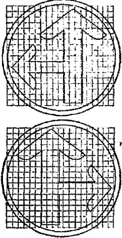
Planche 3. Feux destinés aux conducteurs des bicyclettes et des cyclomoteurs à deux roues.
