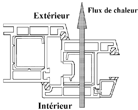
Figure D.4 – Profilé d'encadrement en plastique avec renfort et 3 chambres en série avec le flux thermique
