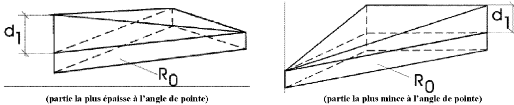
Figure 8 – Éléments de construction avec base triangulaire, composés d'une partie inclinée et d'une partie plane (restante)
