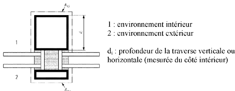
Figure E.2 – Profondeur intérieure des traverses
